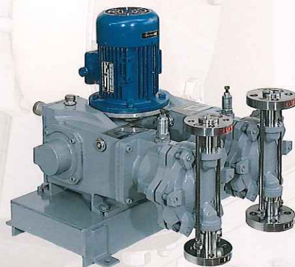
2. pompa a due teste duplex pump pompe duplex
