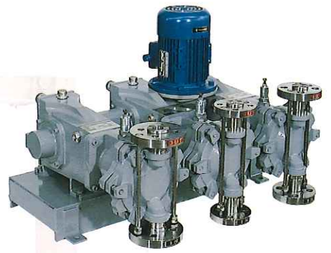
7. gruppo di tre pompe triplex pump groupe triplex
