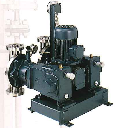
8. pompa duplex 9. con manometro e interruttore d'allarme duplex pump with local and remote alarm pompe duplex avec manomètre et dispositif d'alarme
